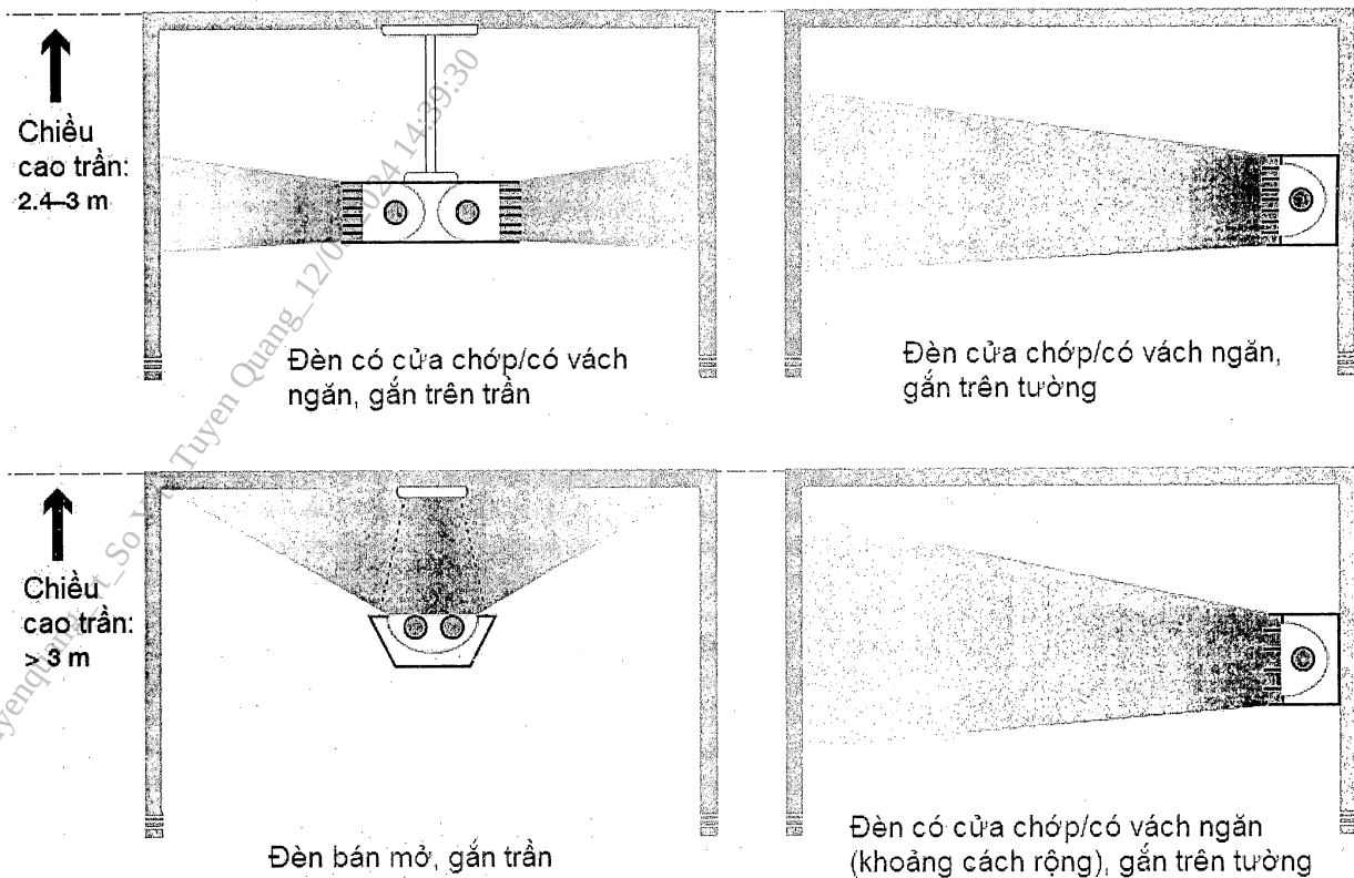
Hình 8: Các loại đèn UV-C gắn trần phù hợp với chiều cao phòng khác nhau 20
