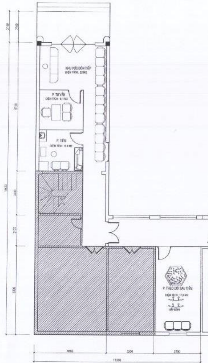
MẶT BẰNG PHÒNG TIỀN
